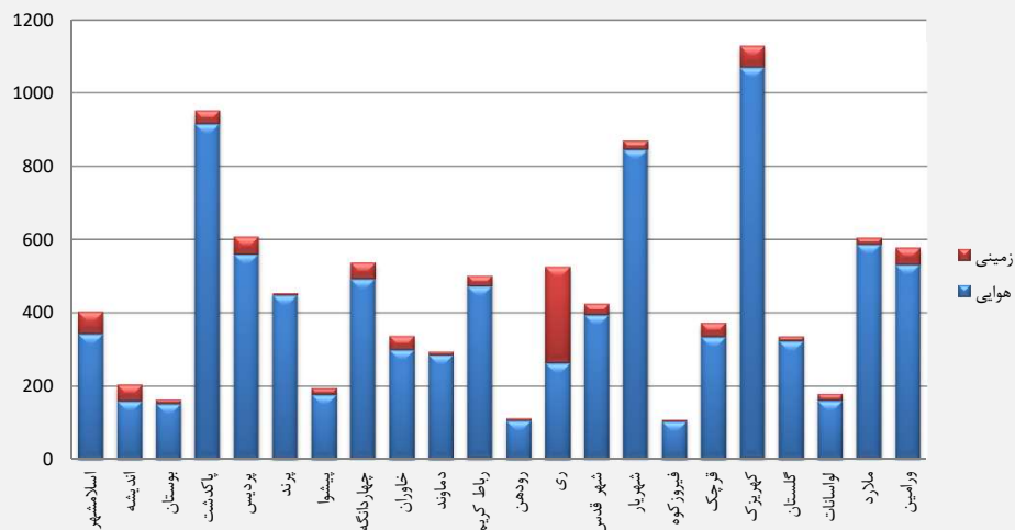
قدرت منصوبه موجود (MVA)
